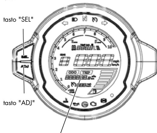
7) Indicatore multifunzione 1
