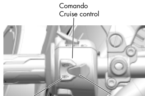
Tasto regolazione velocità ("RES/+" e "SET/-")
